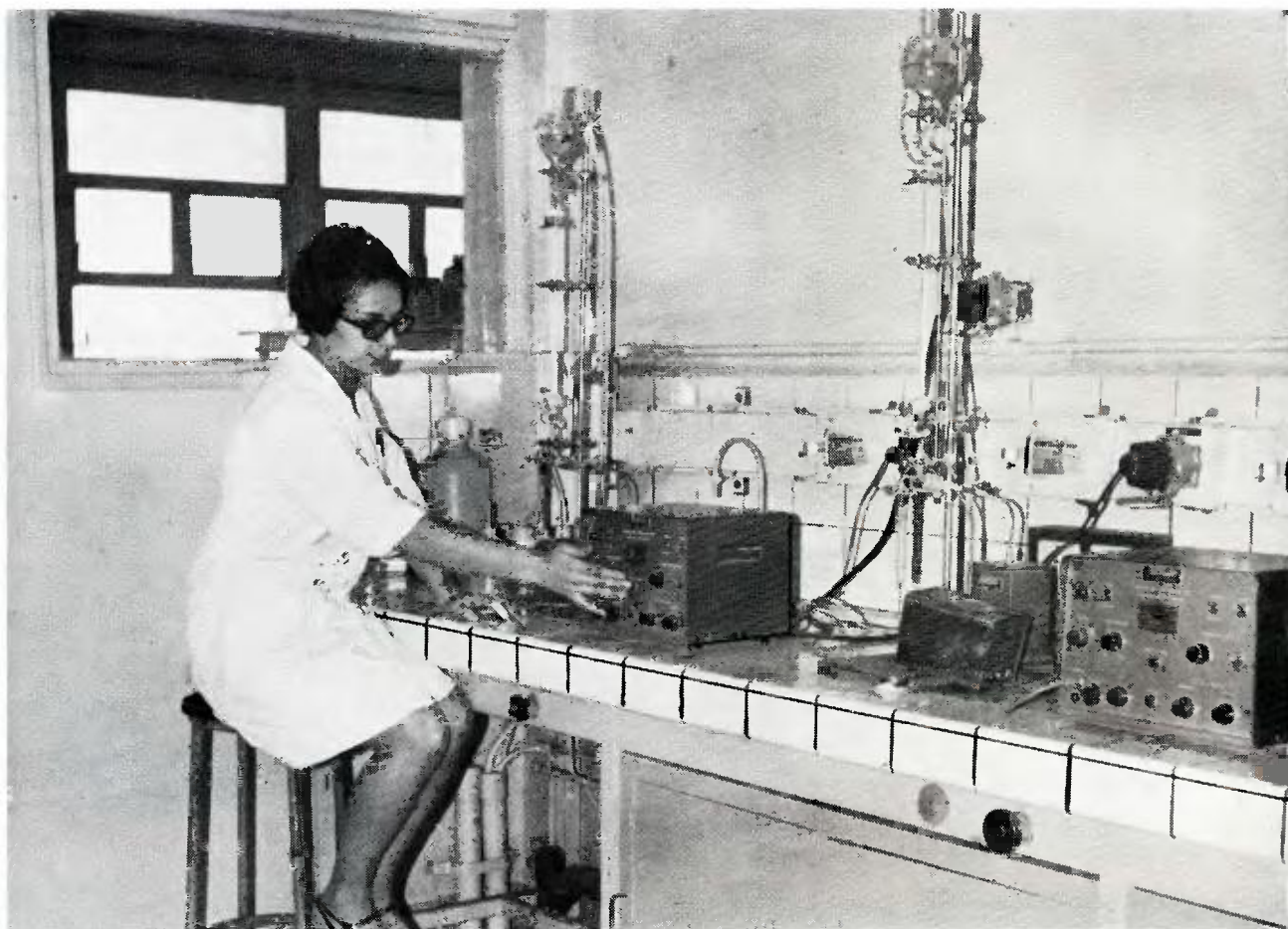
Ἡ κυρία Λούστα ἐνῶ πραγματοποιεῖ ἀνάλυσιν τῆς καθημερινῆς λάσπης στὰ "TITRIMETRE".
