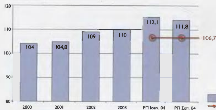
Ρυθμός παραγωγής κολονών (χιλ. τόνου/έτος)
