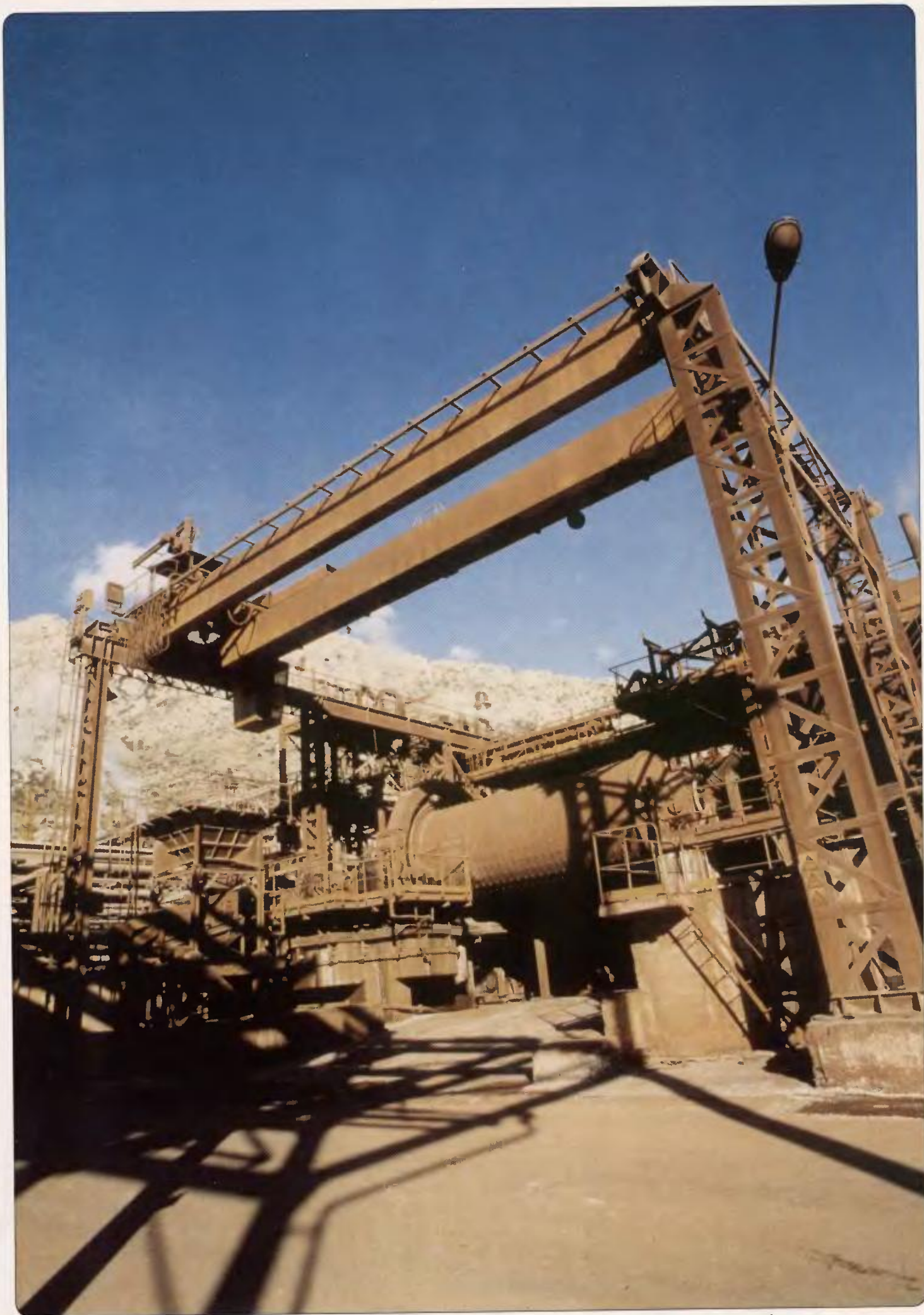
Αποψη του συγκροτήματος άλεσης βωξίτη, στο εργοστάσιο παραγωγής αλουμίνας.
