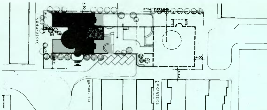
Χωροταξικό σχέδιο του Νηπιακού Σταθμού.
